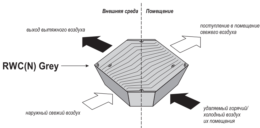
Принцип обмена влажностью
