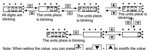
Рис. 4-4 Изменение параметров
